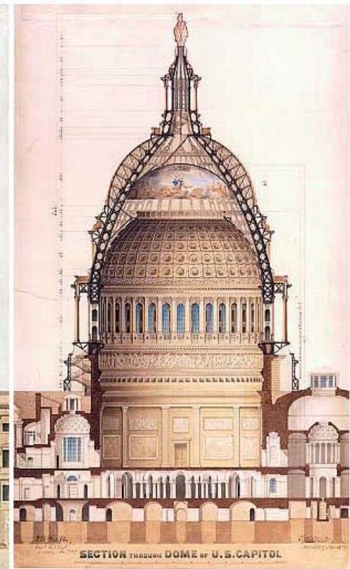
LÄNGSSCHNITT DURCH ROTUNDE UND KUPPEL; ORIGINALZEICHNUNG VON THOMAS USTICK WALTER, 1859
